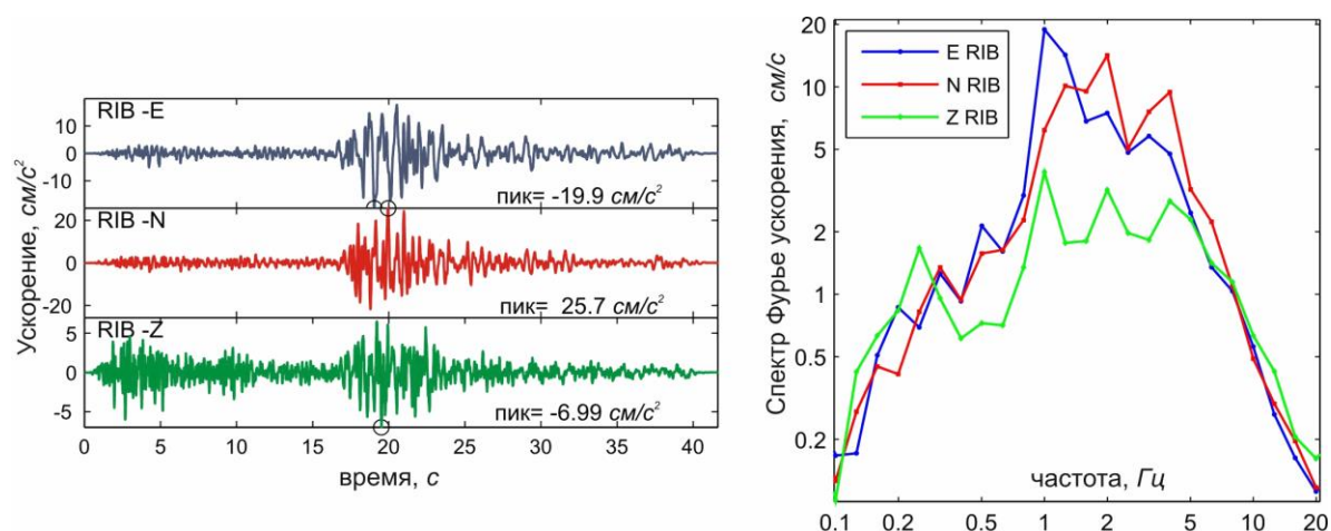
Рис. 8. Три компоненты записи ускорения грунта от землетрясения 30 июля (03 h 56 m ) и сглаженные амплитудные спектры Фурье этих записей
